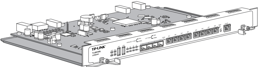
图1-17 TL-SRU7008的外观
